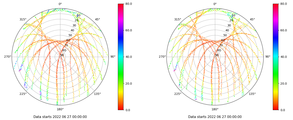
Skyplot for station XIXO. Parameter M1C Data file XIXO00ESP_R_2022178.xtr Skyplot for station XIXO. Parameter M2C Data file XIXO00ESP_R_2022178.xtr
