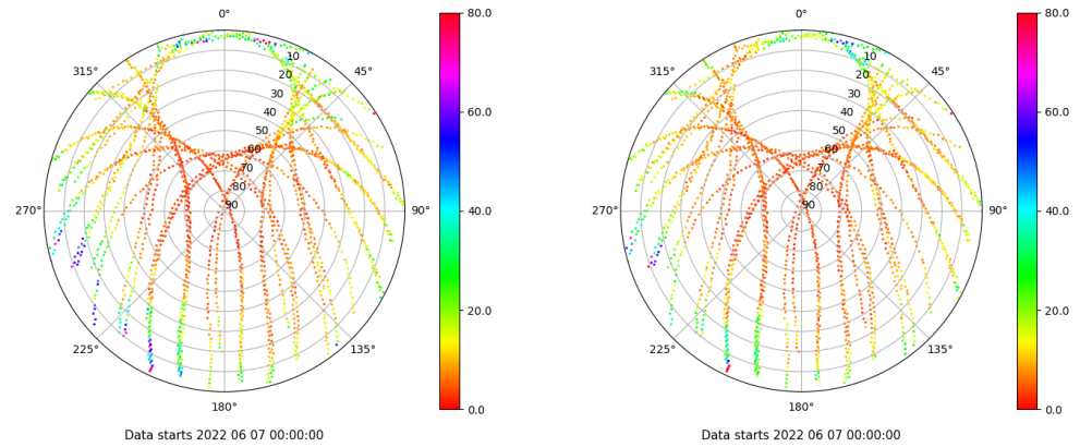
Skyplot for station XIXO. Parameter M1C Data file XIXO00ESP_R_2022158.xtr Skyplot for station XIXO. Parameter M2C Data file XIXO00ESP_R_2022158.xtr
