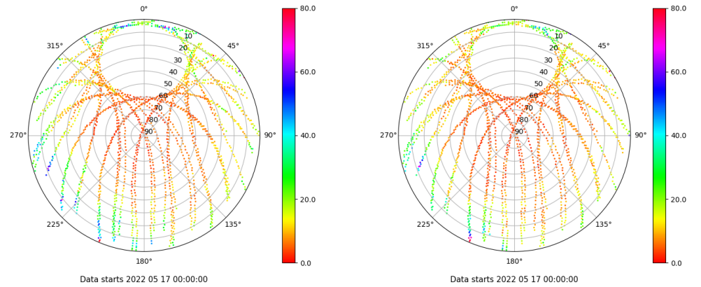
Skyplot for station XIXO. Parameter M1C Data file XIXO00ESP_R_2022137.xtr Skyplot for station XIXO. Parameter M2C Data file XIXO00ESP_R_2022137.xtr
