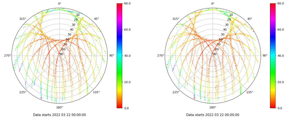
Skyplot for station XIXO. Parameter M1C Data file XIXO00ESP_R_2022081.xtr Skyplot for station XIXO. Parameter M2C Data file XIXO00ESP_R_2022081.xtr
