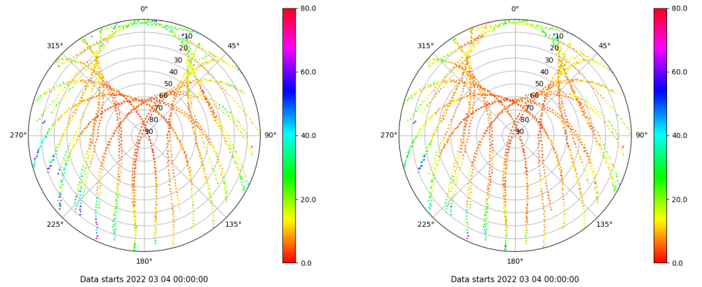
Skyplot for station XIXO. Parameter M1C Data file XIXO00ESP_R_2022063.xtr Skyplot for station XIXO. Parameter M2C Data file XIXO00ESP_R_2022063.xtr
