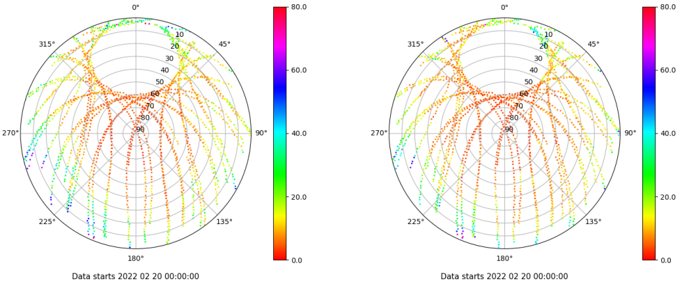
Skyplot for station XIXO. Parameter M1C Data file XIXO00ESP_R_2022051.xtr Skyplot for station XIXO. Parameter M2C Data file XIXO00ESP_R_2022051.xtr
