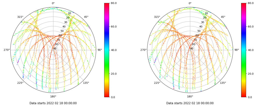
Skyplot for station XIXO. Parameter M1C Data file XIXO00ESP_R_2022049.xtr Skyplot for station XIXO. Parameter M2C Data file XIXO00ESP_R_2022049.xtr
