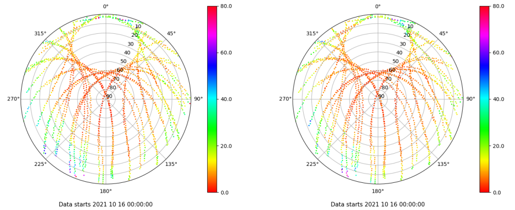
Skyplot for station XIXO. Parameter M1C Data file XIXO00ESP_R_2021289.xtr Skyplot for station XIXO. Parameter M2C Data file XIXO00ESP_R_2021289.xtr
