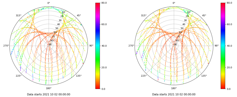
Skyplot for station XIXO. Parameter M1C Data file XIXO00ESP_R_2021275.xtr Skyplot for station XIXO. Parameter M2C Data file XIXO00ESP_R_2021275.xtr
