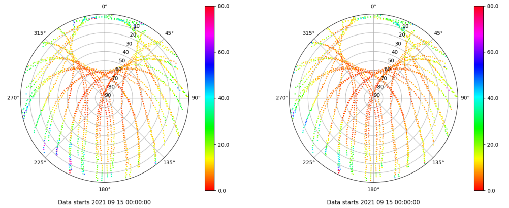
Skyplot for station XIXO. Parameter M1C Data file XIXO00ESP_R_2021258.xtr Skyplot for station XIXO. Parameter M2C Data file XIXO00ESP_R_2021258.xtr
