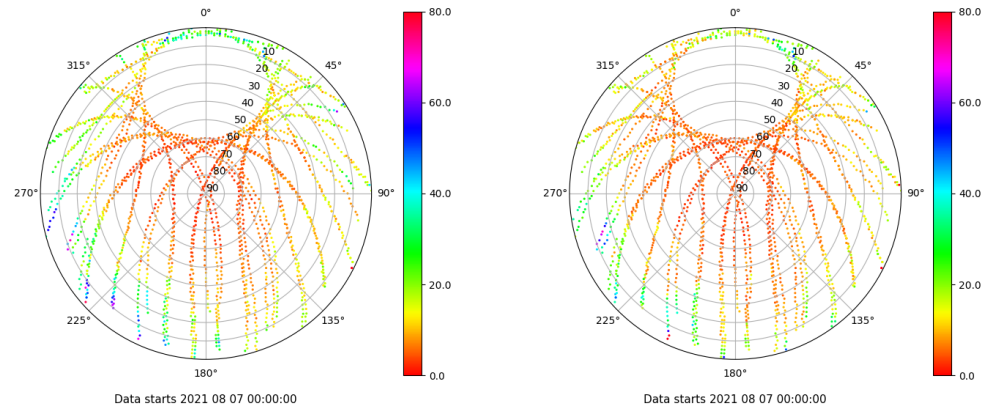
Skyplot for station XIXO. Parameter M1C Data file XIXO00ESP_R_2021219.xtr Skyplot for station XIXO. Parameter M2C Data file XIXO00ESP_R_2021219.xtr
