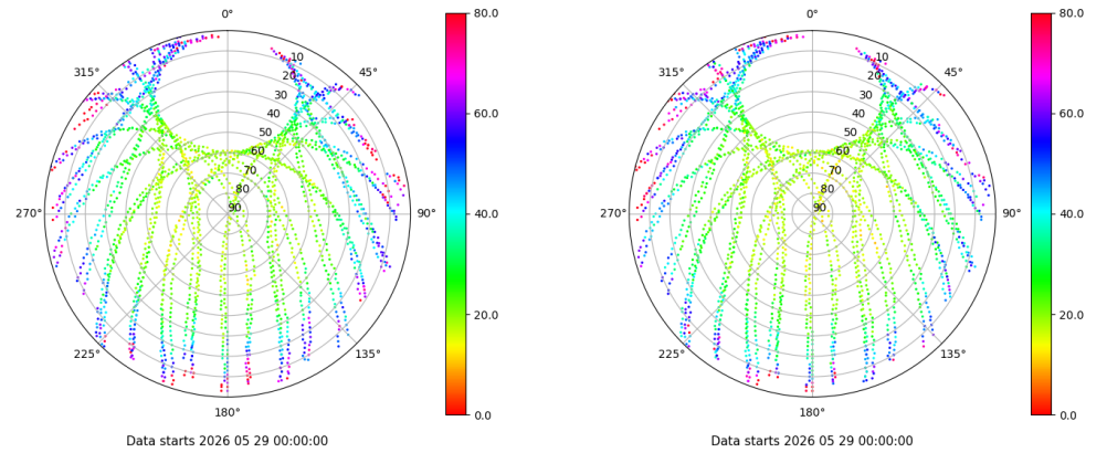
Skyplot for station VIGO. Parameter M1C Data file VIGO00ESP_R_2026149.xtr Skyplot for station VIGO. Parameter M2C Data file VIGO00ESP_R_2026149.xtr
