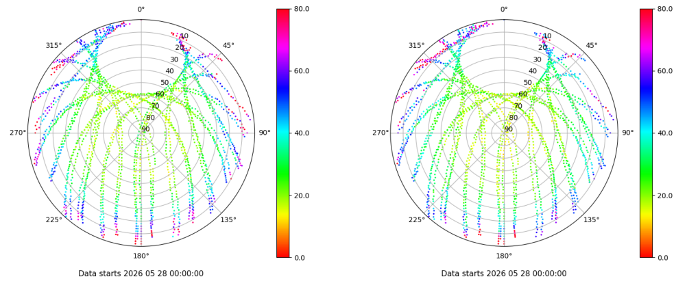
Skyplot for station VIGO. Parameter M1C Data file VIGO00ESP_R_2026148.xtr Skyplot for station VIGO. Parameter M2C Data file VIGO00ESP_R_2026148.xtr
