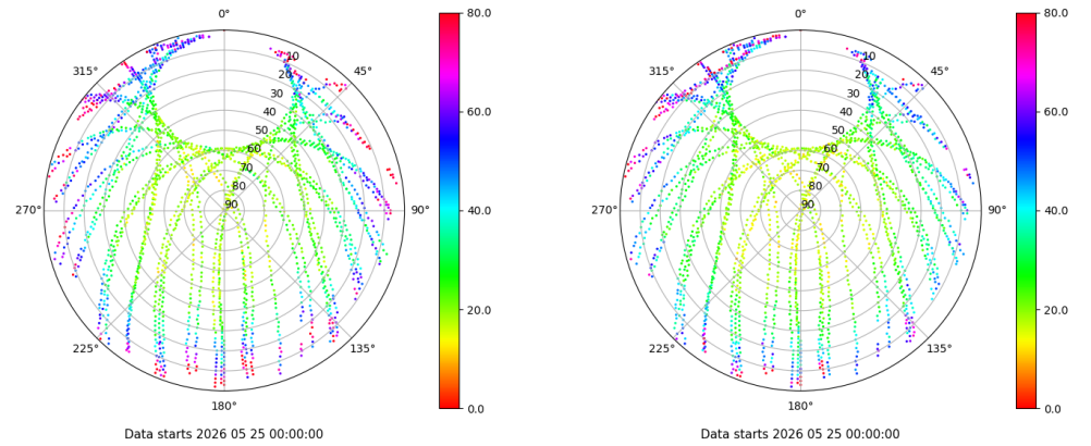
Skyplot for station VIGO. Parameter M1C Data file VIGO00ESP_R_2026145.xtr Skyplot for station VIGO. Parameter M2C Data file VIGO00ESP_R_2026145.xtr
