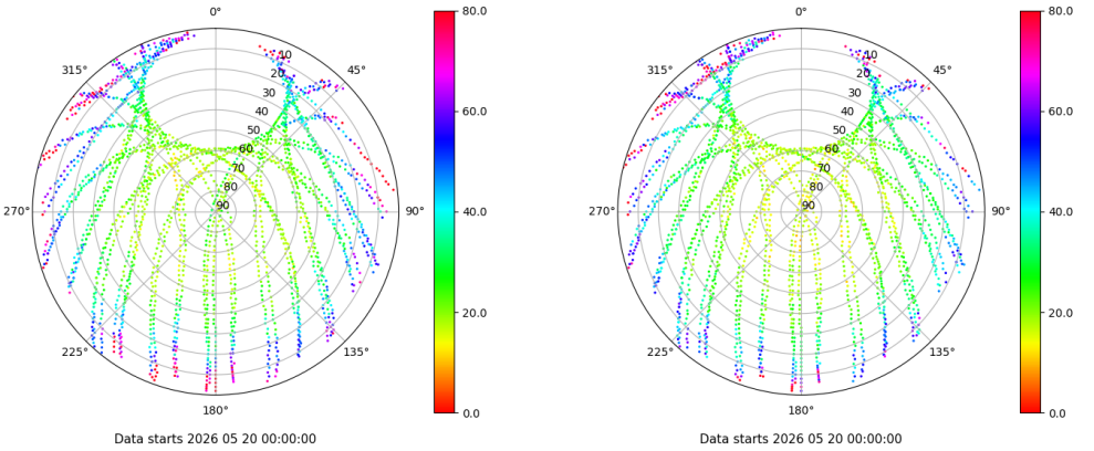
Skyplot for station VIGO. Parameter M1C Data file VIGO00ESP_R_2026140.xtr Skyplot for station VIGO. Parameter M2C Data file VIGO00ESP_R_2026140.xtr
