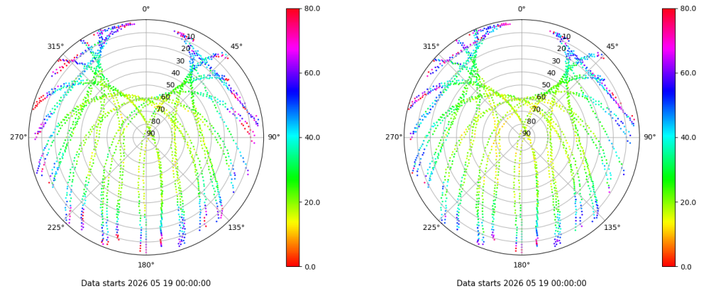
Skyplot for station VIGO. Parameter M1C Data file VIGO00ESP_R_2026139.xtr Skyplot for station VIGO. Parameter M2C Data file VIGO00ESP_R_2026139.xtr
