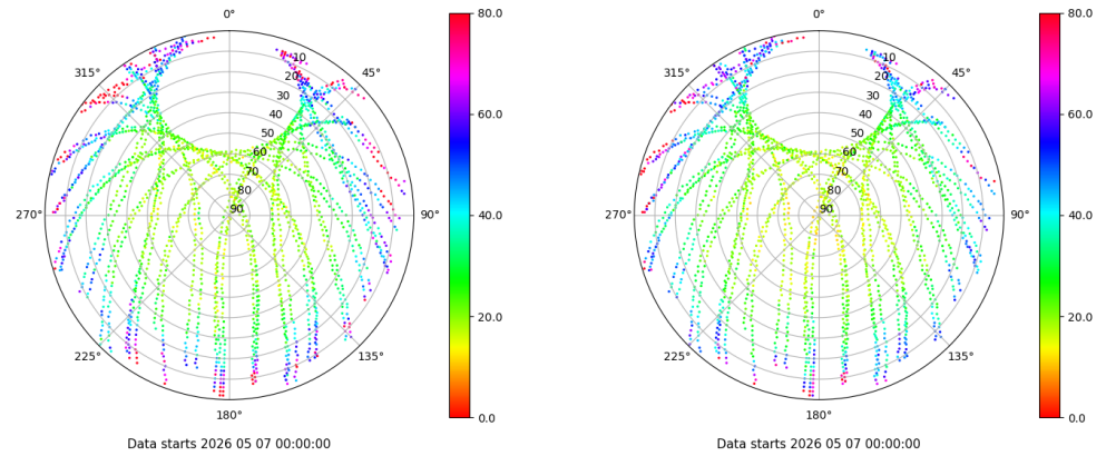
Skyplot for station VIGO. Parameter M1C Data file VIGO00ESP_R_2026127.xtr Skyplot for station VIGO. Parameter M2C Data file VIGO00ESP_R_2026127.xtr
