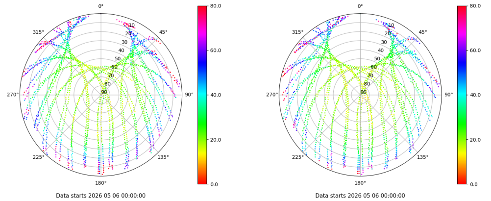
Skyplot for station VIGO. Parameter M1C Data file VIGO00ESP_R_2026126.xtr Skyplot for station VIGO. Parameter M2C Data file VIGO00ESP_R_2026126.xtr
