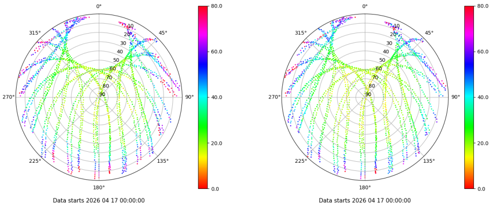
Skyplot for station VIGO. Parameter M1C Data file VIGO00ESP_R_2026107.xtr Skyplot for station VIGO. Parameter M2C Data file VIGO00ESP_R_2026107.xtr
