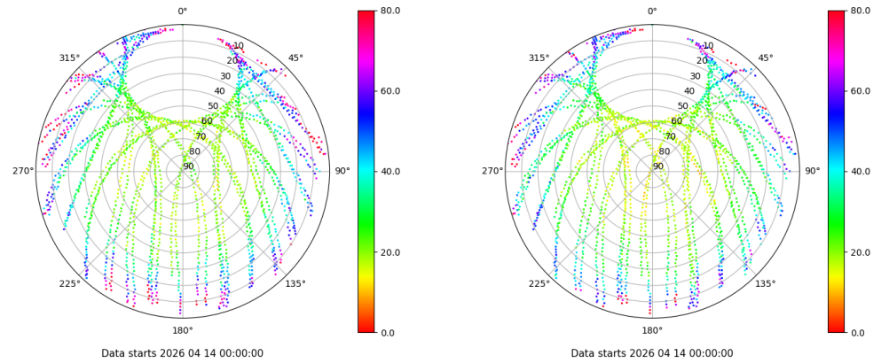
Skyplot for station VIGO. Parameter M1C Data file VIGO00ESP_R_2026104.xtr Skyplot for station VIGO. Parameter M2C Data file VIGO00ESP_R_2026104.xtr
