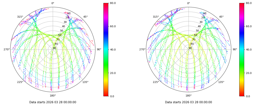
Skyplot for station VIGO. Parameter M1C Data file VIGO00ESP_R_2026087.xtr Skyplot for station VIGO. Parameter M2C Data file VIGO00ESP_R_2026087.xtr
