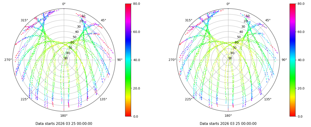
Skyplot for station VIGO. Parameter M1C Data file VIGO00ESP_R_2026084.xtr Skyplot for station VIGO. Parameter M2C Data file VIGO00ESP_R_2026084.xtr
