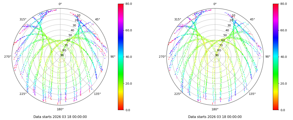
Skyplot for station VIGO. Parameter M1C Data file VIGO00ESP_R_2026077.xtr Skyplot for station VIGO. Parameter M2C Data file VIGO00ESP_R_2026077.xtr
