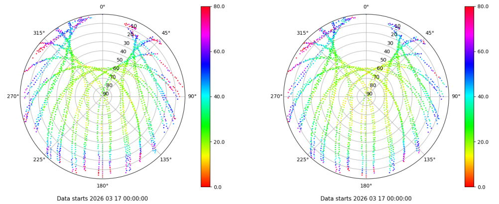
Skyplot for station VIGO. Parameter M1C Data file VIGO00ESP_R_2026076.xtr Skyplot for station VIGO. Parameter M2C Data file VIGO00ESP_R_2026076.xtr
