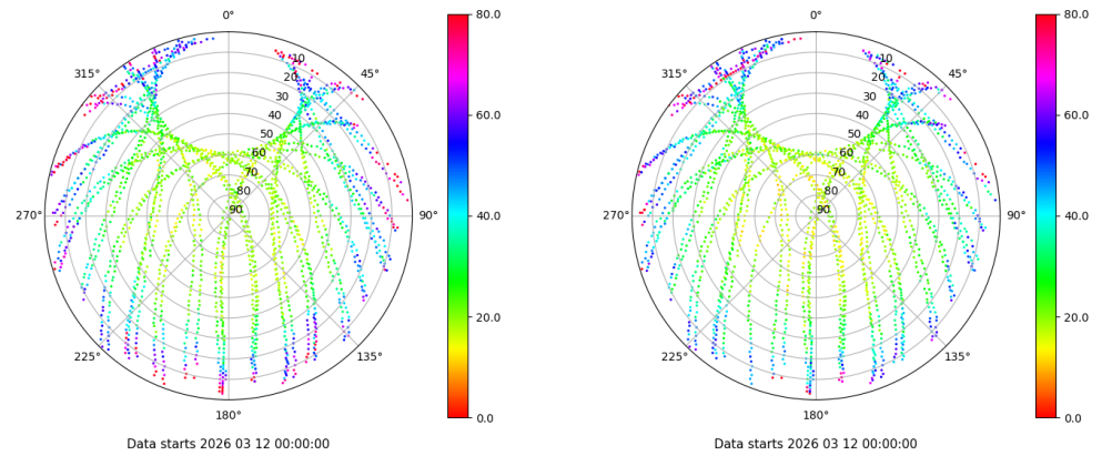
Skyplot for station VIGO. Parameter M1C Data file VIGO00ESP_R_2026071.xtr Skyplot for station VIGO. Parameter M2C Data file VIGO00ESP_R_2026071.xtr
