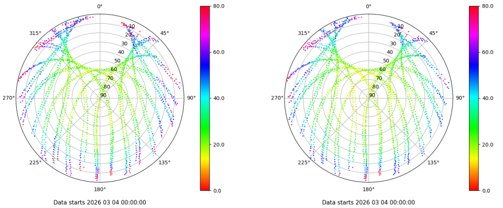
Skyplot for station VIGO. Parameter M1C Data file VIGO00ESP_R_2026063.xtr Skyplot for station VIGO. Parameter M2C Data file VIGO00ESP_R_2026063.xtr
