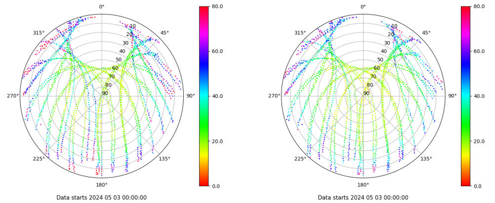
Skyplot for station VIGO. Parameter M1C Data file VIGO00ESP_R_2024124.xtr Skyplot for station VIGO. Parameter M2C Data file VIGO00ESP_R_2024124.xtr
