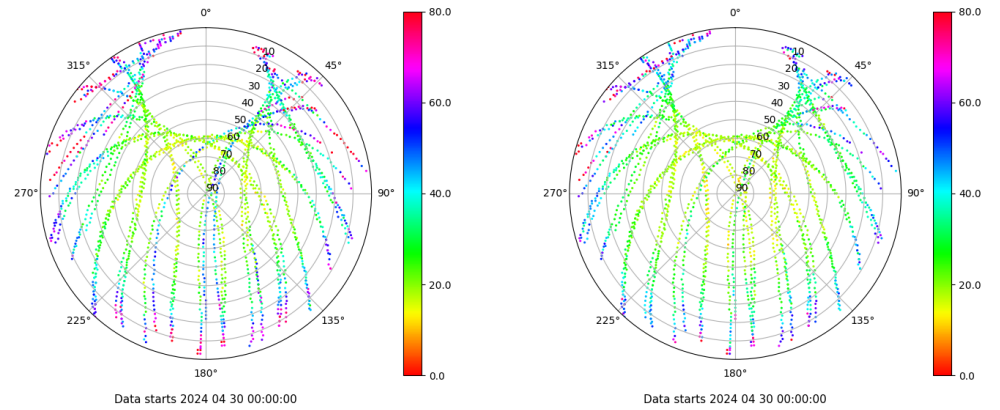
Skyplot for station VIGO. Parameter M1C Data file VIGO00ESP_R_2024121.xtr Skyplot for station VIGO. Parameter M2C Data file VIGO00ESP_R_2024121.xtr
