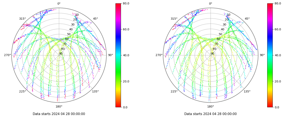
Skyplot for station VIGO. Parameter M1C Data file VIGO00ESP_R_2024119.xtr Skyplot for station VIGO. Parameter M2C Data file VIGO00ESP_R_2024119.xtr
