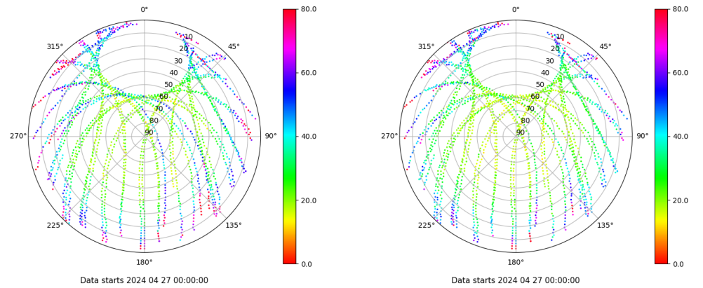
Skyplot for station VIGO. Parameter M1C Data file VIGO00ESP_R_2024118.xtr Skyplot for station VIGO. Parameter M2C Data file VIGO00ESP_R_2024118.xtr
