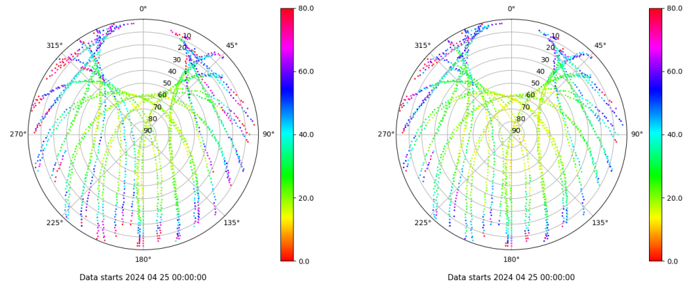
Skyplot for station VIGO. Parameter M1C Data file VIGO00ESP_R_2024116.xtr Skyplot for station VIGO. Parameter M2C Data file VIGO00ESP_R_2024116.xtr
