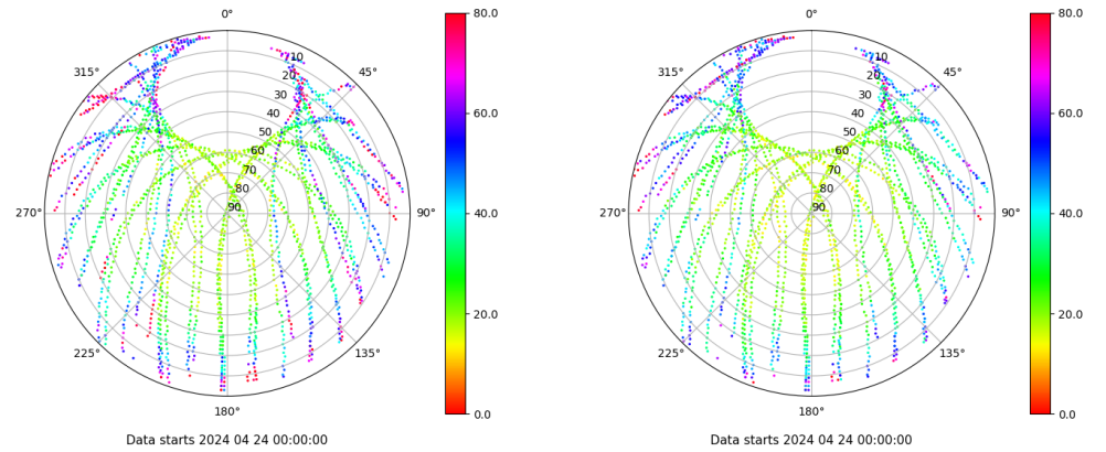
Skyplot for station VIGO. Parameter M1C Data file VIGO00ESP_R_2024115.xtr Skyplot for station VIGO. Parameter M2C Data file VIGO00ESP_R_2024115.xtr
