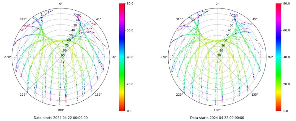
Skyplot for station VIGO. Parameter M1C Data file VIGO00ESP_R_2024113.xtr Skyplot for station VIGO. Parameter M2C Data file VIGO00ESP_R_2024113.xtr
