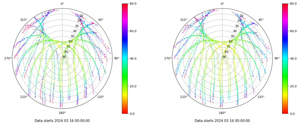
Skyplot for station VIGO. Parameter M1C Data file VIGO00ESP_R_2024076.xtr Skyplot for station VIGO. Parameter M2C Data file VIGO00ESP_R_2024076.xtr
