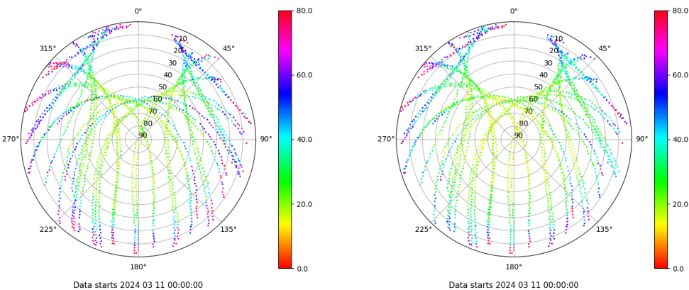
Skyplot for station VIGO. Parameter M1C Data file VIGO00ESP_R_2024071.xtr Skyplot for station VIGO. Parameter M2C Data file VIGO00ESP_R_2024071.xtr
