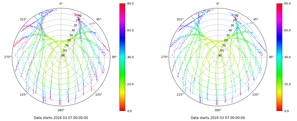
Skyplot for station VIGO. Parameter M1C Data file VIGO00ESP_R_2024067.xtr Skyplot for station VIGO. Parameter M2C Data file VIGO00ESP_R_2024067.xtr
