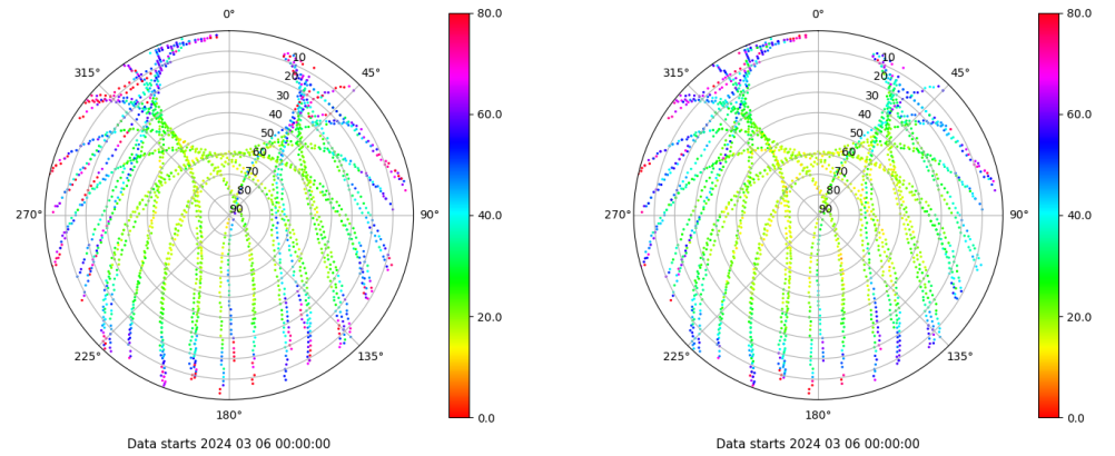
Skyplot for station VIGO. Parameter M1C Data file VIGO00ESP_R_2024066.xtr Skyplot for station VIGO. Parameter M2C Data file VIGO00ESP_R_2024066.xtr
