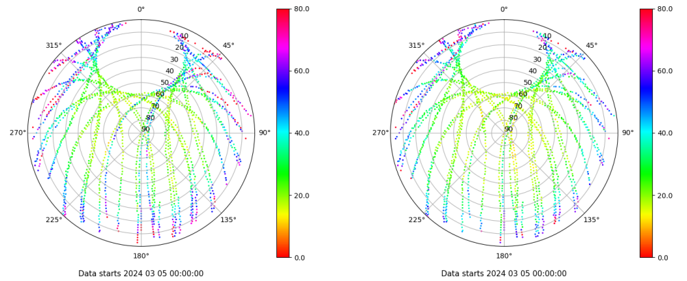
Skyplot for station VIGO. Parameter M1C Data file VIGO00ESP_R_2024065.xtr Skyplot for station VIGO. Parameter M2C Data file VIGO00ESP_R_2024065.xtr
