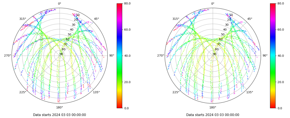
Skyplot for station VIGO. Parameter M1C Data file VIGO00ESP_R_2024063.xtr Skyplot for station VIGO. Parameter M2C Data file VIGO00ESP_R_2024063.xtr
