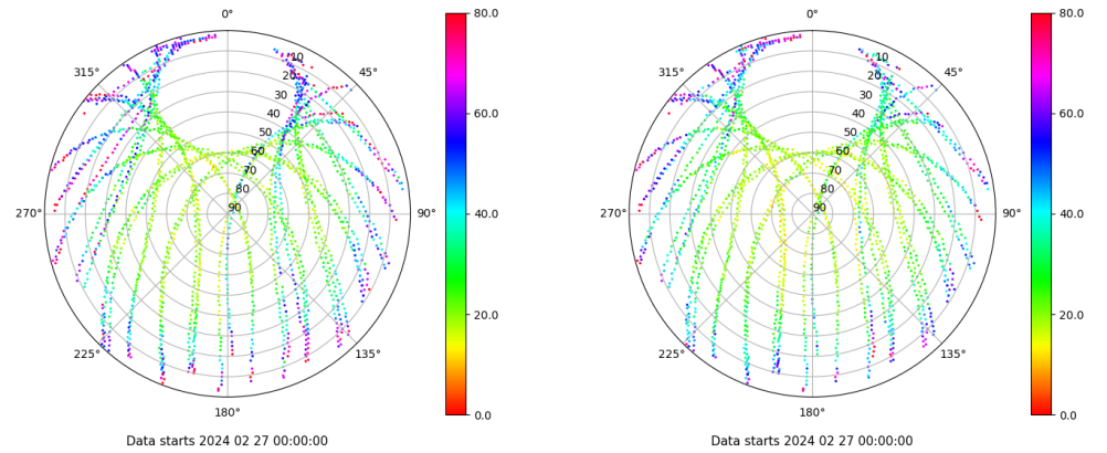
Skyplot for station VIGO. Parameter M1C Data file VIGO00ESP_R_2024058.xtr Skyplot for station VIGO. Parameter M2C Data file VIGO00ESP_R_2024058.xtr
