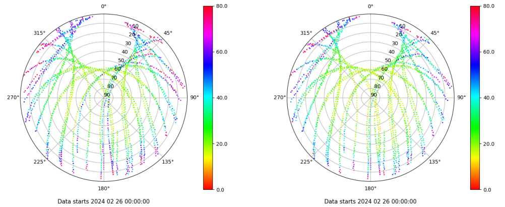
Skyplot for station VIGO. Parameter M1C Data file VIGO00ESP_R_2024057.xtr Skyplot for station VIGO. Parameter M2C Data file VIGO00ESP_R_2024057.xtr
