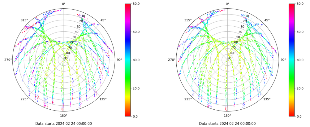
Skyplot for station VIGO. Parameter M1C Data file VIGO00ESP_R_2024055.xtr Skyplot for station VIGO. Parameter M2C Data file VIGO00ESP_R_2024055.xtr
