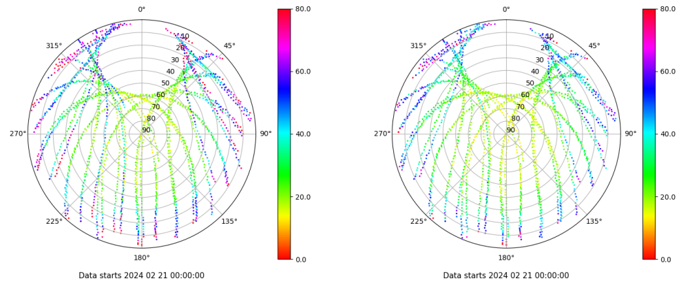
Skyplot for station VIGO. Parameter M1C Data file VIGO00ESP_R_2024052.xtr Skyplot for station VIGO. Parameter M2C Data file VIGO00ESP_R_2024052.xtr
