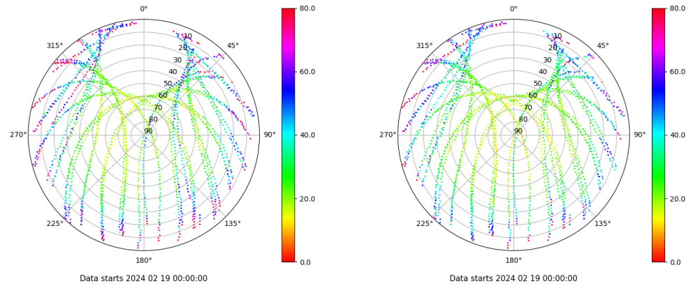
Skyplot for station VIGO. Parameter M1C Data file VIGO00ESP_R_2024050.xtr Skyplot for station VIGO. Parameter M2C Data file VIGO00ESP_R_2024050.xtr
