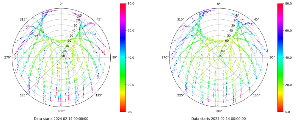
Skyplot for station VIGO. Parameter M1C Data file VIGO00ESP_R_2024045.xtr Skyplot for station VIGO. Parameter M2C Data file VIGO00ESP_R_2024045.xtr
