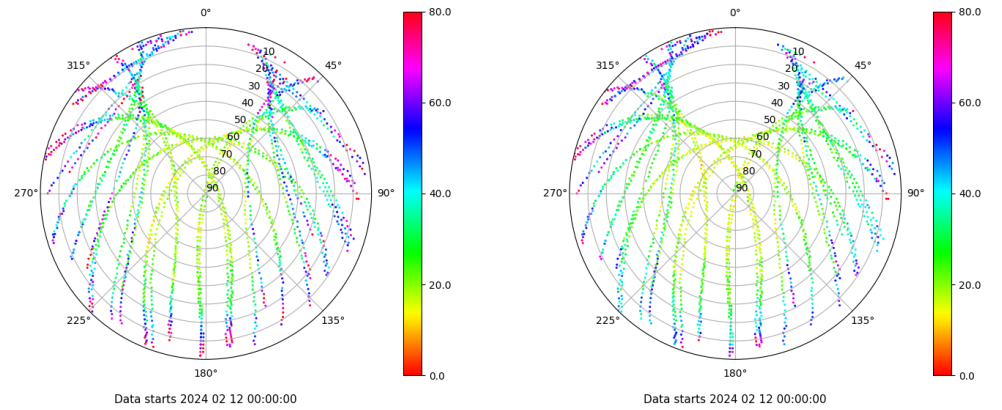
Skyplot for station VIGO. Parameter M1C Data file VIGO00ESP_R_2024043.xtr Skyplot for station VIGO. Parameter M2C Data file VIGO00ESP_R_2024043.xtr
