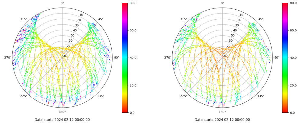
Skyplot for station VIGO. Parameter M1C Data file VIGO00ESP_R_2024043.xtr Skyplot for station VIGO. Parameter M2X Data file VIGO00ESP_R_2024043.xtr
