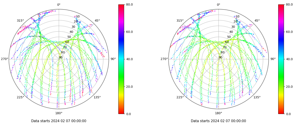
Skyplot for station VIGO. Parameter M1C Data file VIGO00ESP_R_2024038.xtr Skyplot for station VIGO. Parameter M2C Data file VIGO00ESP_R_2024038.xtr
