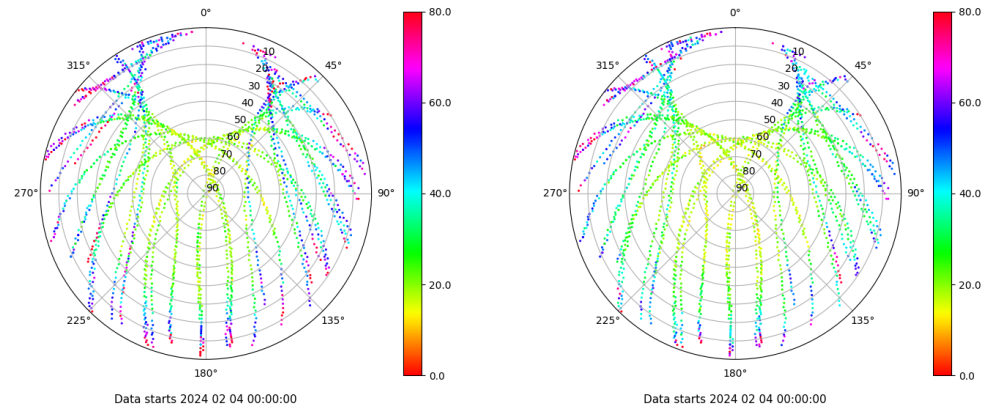
Skyplot for station VIGO. Parameter M1C Data file VIGO00ESP_R_2024035.xtr Skyplot for station VIGO. Parameter M2C Data file VIGO00ESP_R_2024035.xtr
