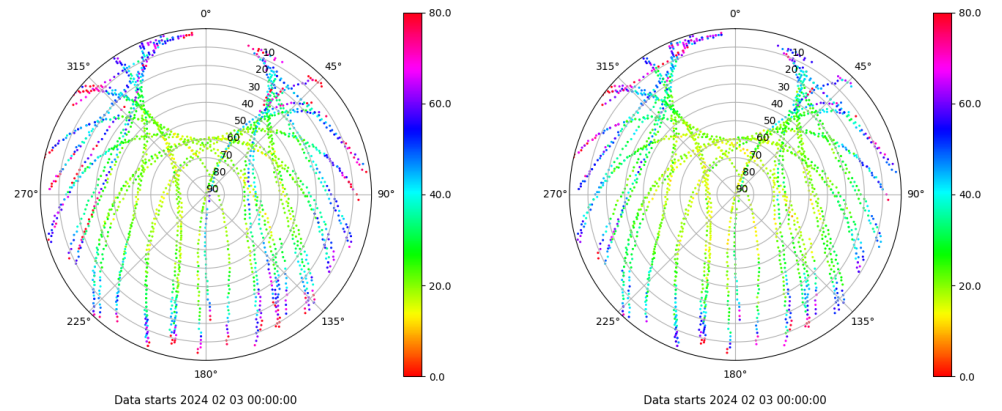
Skyplot for station VIGO. Parameter M1C Data file VIGO00ESP_R_2024034.xtr Skyplot for station VIGO. Parameter M2C Data file VIGO00ESP_R_2024034.xtr
