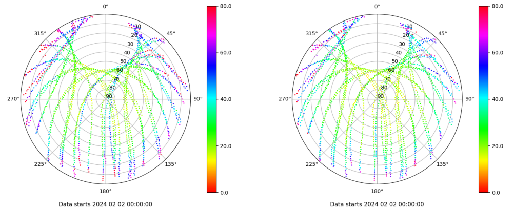
Skyplot for station VIGO. Parameter M1C Data file VIGO00ESP_R_2024033.xtr Skyplot for station VIGO. Parameter M2C Data file VIGO00ESP_R_2024033.xtr
